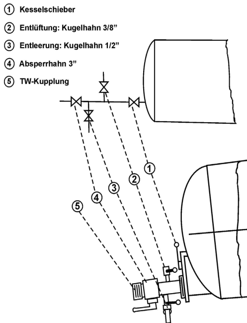
Probenahmeverrichtung an Vakuum-Tankwagen
